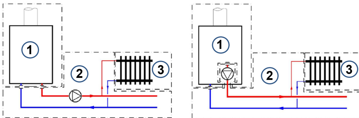
Slika 3-7 Podsustavi centralnog sustava grijanja
