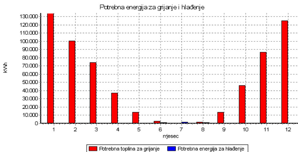
Slika 5-3 Primjer prikaza potrebne toplinske energije za grijanje i hlađenje
