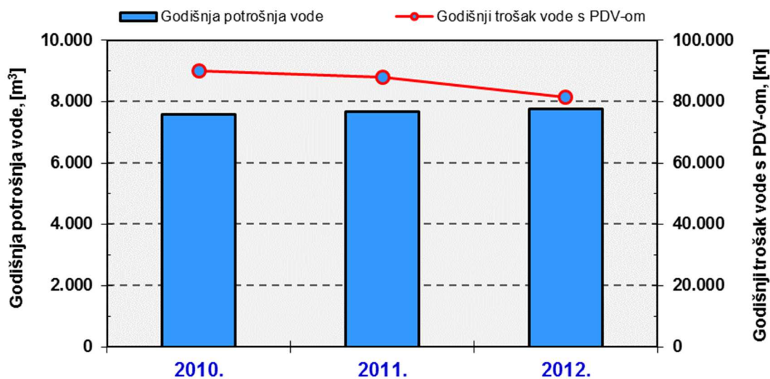
Slika 4-12 Ukupna godišnja potrošnja vode s pripadajućim troškovima za tri uzastopne godine 2010., 2011. i 2012. – hotel
