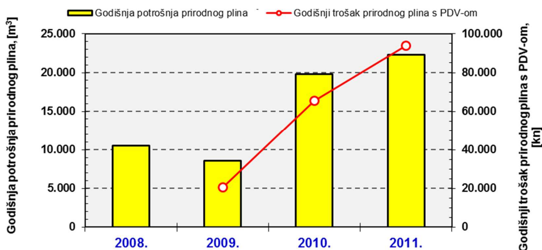
Slika 4-10 Ukupna godišnja potrošnja prirodnog plina s pripadajućim troškovima za četiri uzastopne godine 2008., 2009., 2010. i 2011. – UREDSKA ZGRADA
