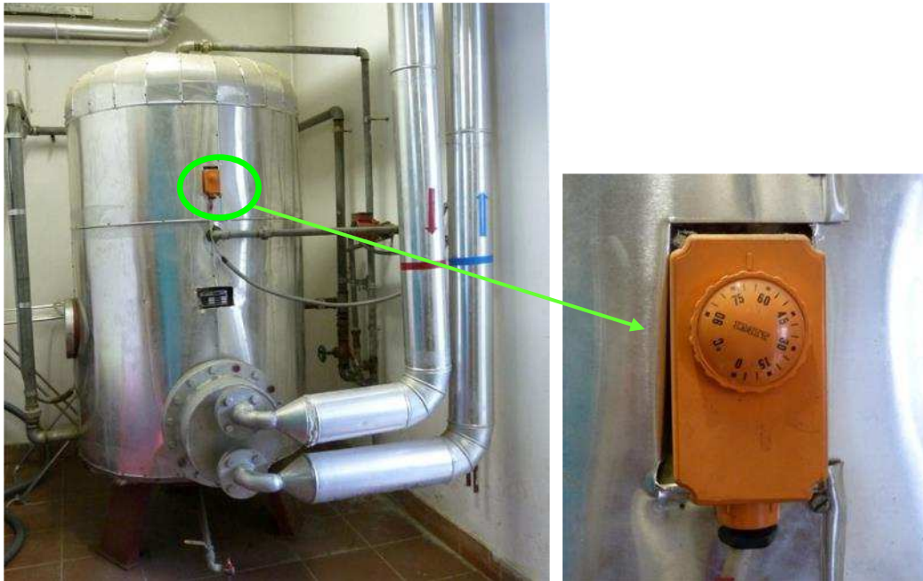
Slika 3-16 Spremnik potrošne tople vode volumena 1.000 litara za potrebe kuhinje
