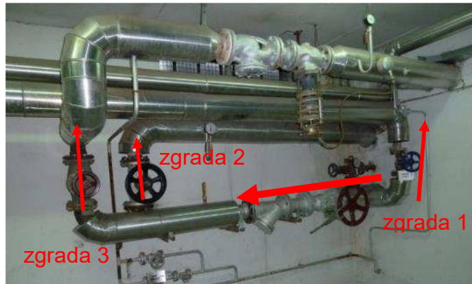
Slika 3-38 Podstava razvoda pare u zgradi
