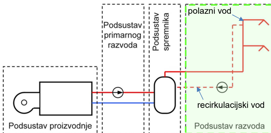
Slika 3-17 Uobičajeni izvori toplinske energije centralnog sustava grijanja
