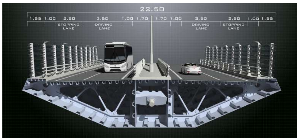
Slika 9. Konstrukcija rasponskog sklopa s prometnim plohami
