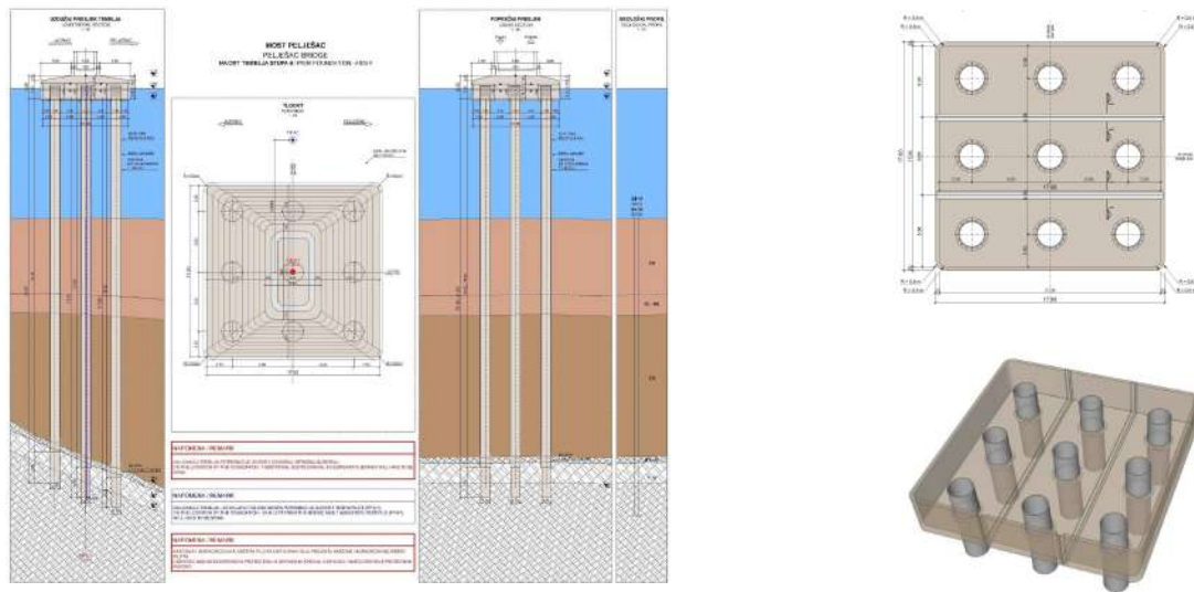
Slika 12. Temeljenje stupova S3, S4, S11, S12
